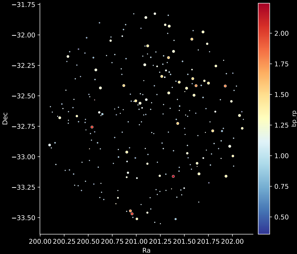
GALAH DR4 Field: [2930] Stars: 262
