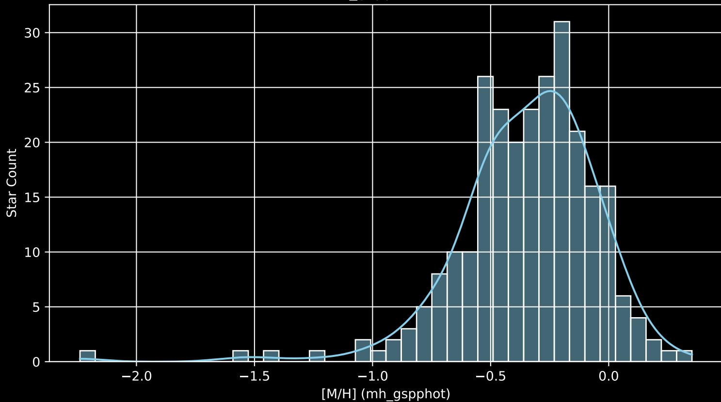
GALAH DR4 Field: [2930] [M/H] (mh_gspphot) (n= 261)
