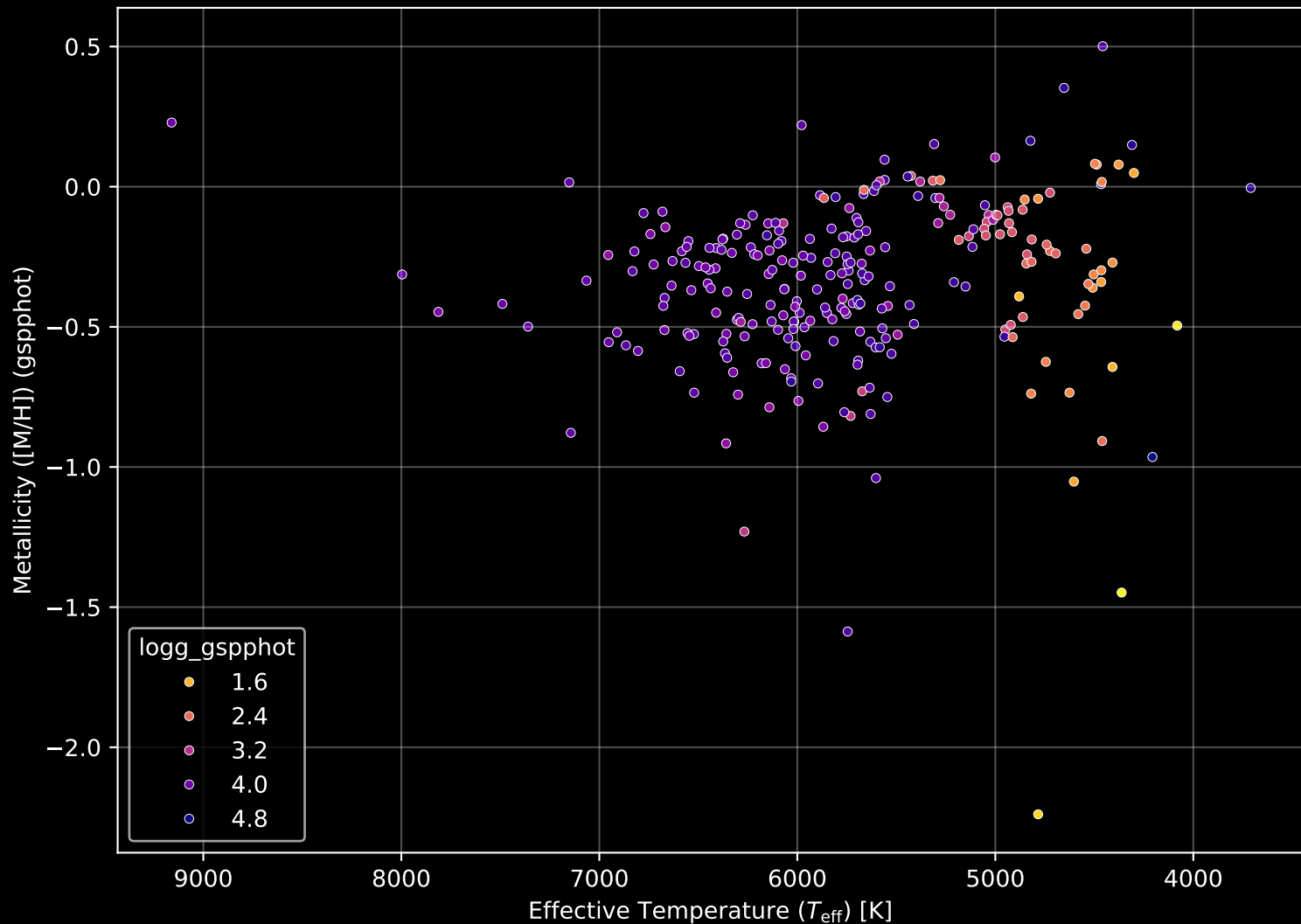
GALAH DR4 Field: [2930] Stellar Population Parameters (n= 262)
