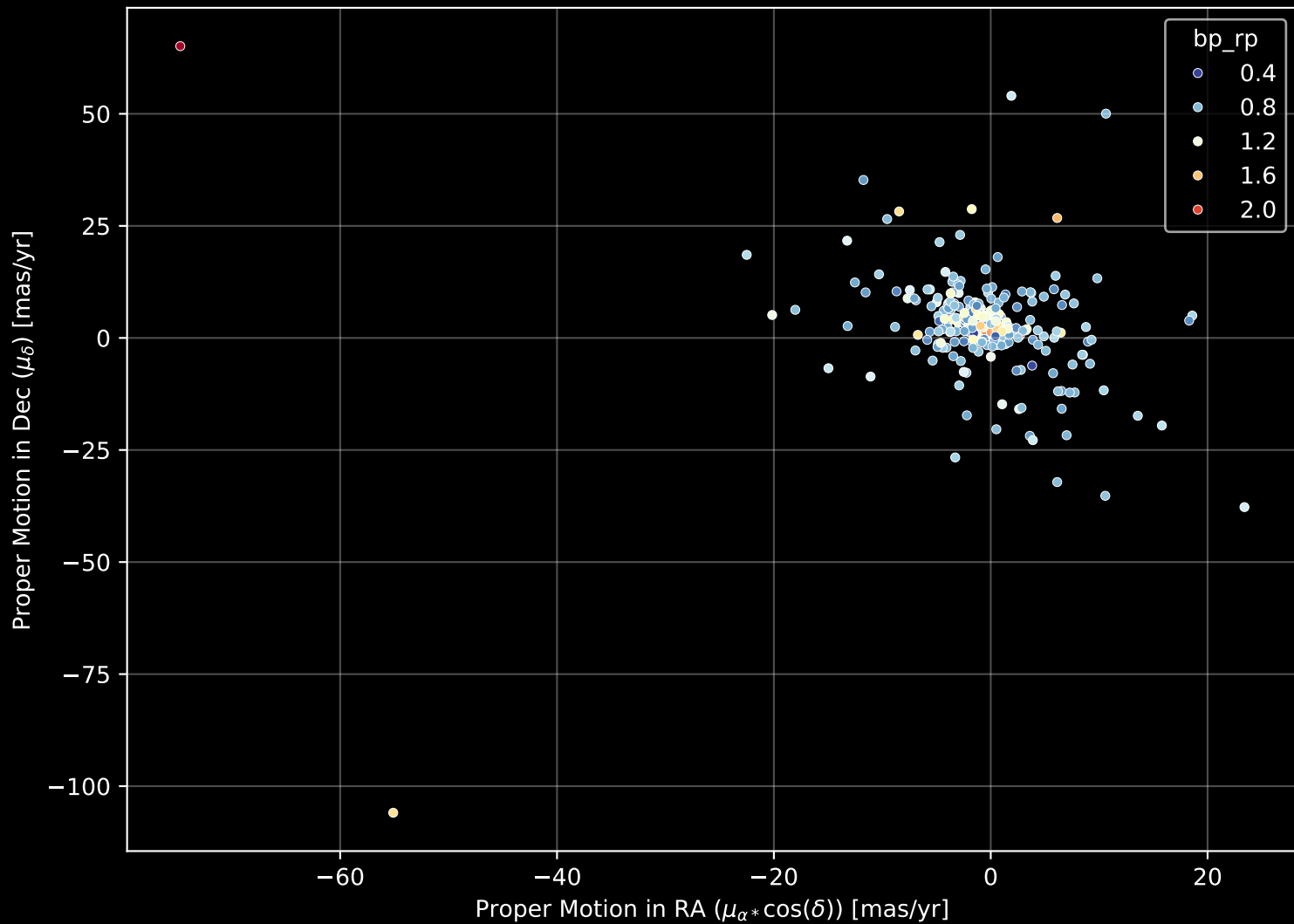
GALAH DR4 Field: [2930] Proper Motion Diagram (n= 262)
