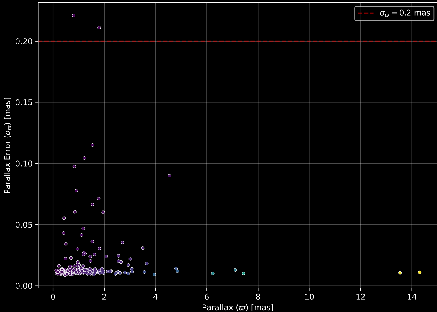
GALAH DR4 Field: [2930] Parallax Quality (n= 262)
